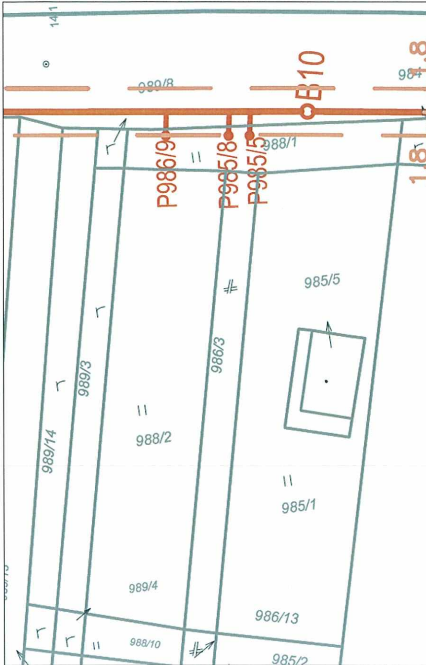
Príloha: Snímka PD so zakresom trás kanalizačného potrubia
