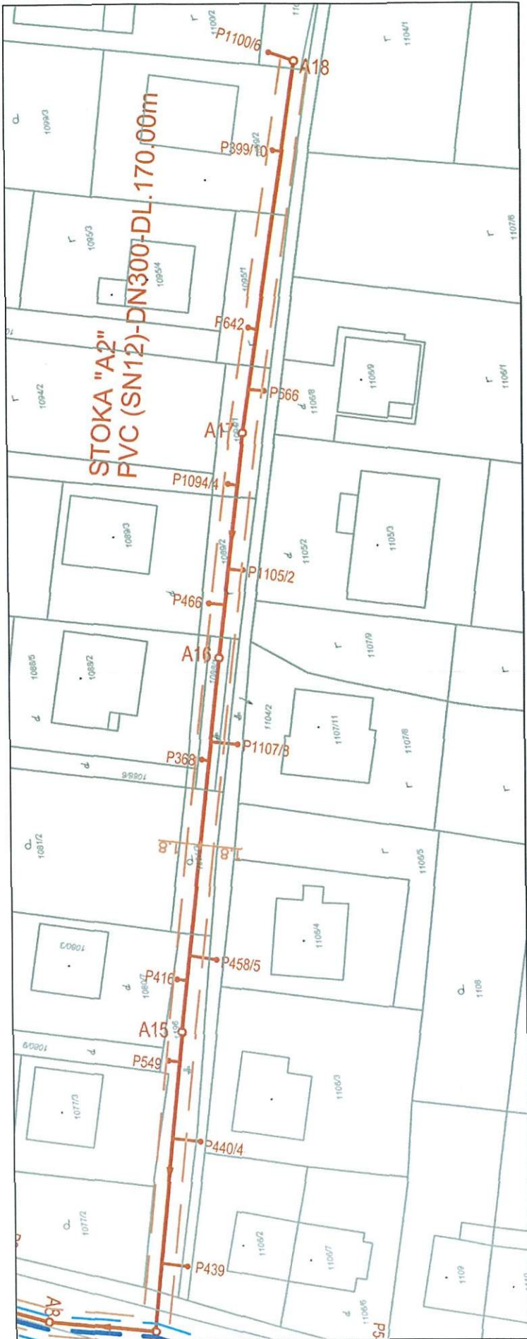
Príloha: Snímka PD so zákresom trás kanalizačného potrubia
