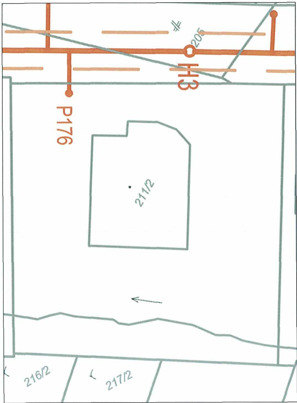
Príloha: Snímka PD so zákresom trás kanalizačného potrubia
